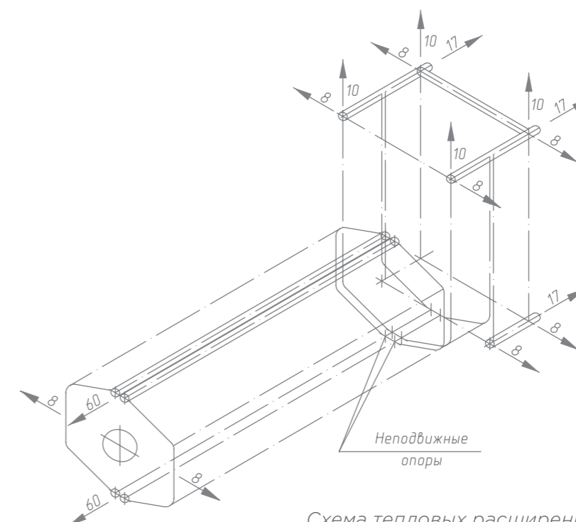
Схема тепловых расширений в мм.
