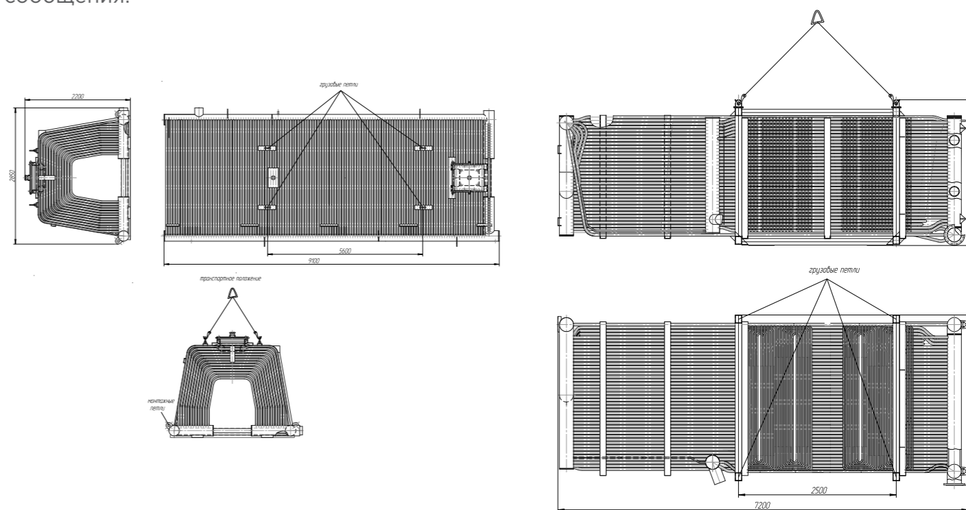
Блоки топочные установочное положение
