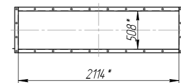
Выход газов
